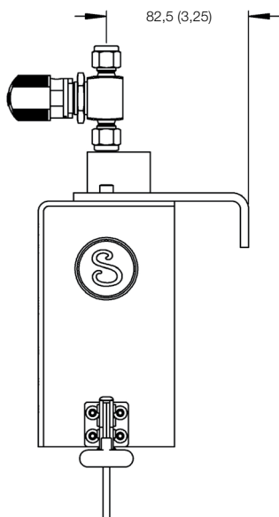
Vue de côté – Configuration droite
