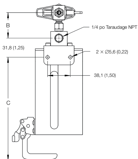
Vue de derrière – Configuration en angle
