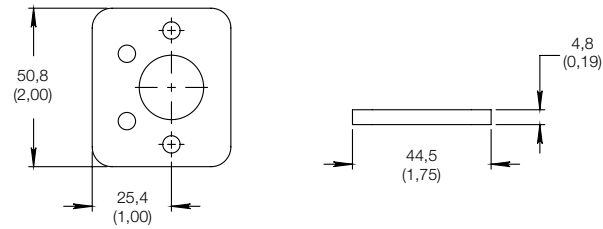
Adaptateur réceptacle/armoire (Référence : 304-GSV-MBK-S)
