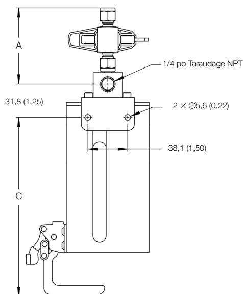
Vue de derrière – Configuration droite
