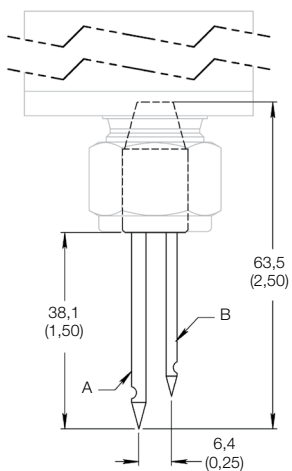
Aiguilles côte à côte
