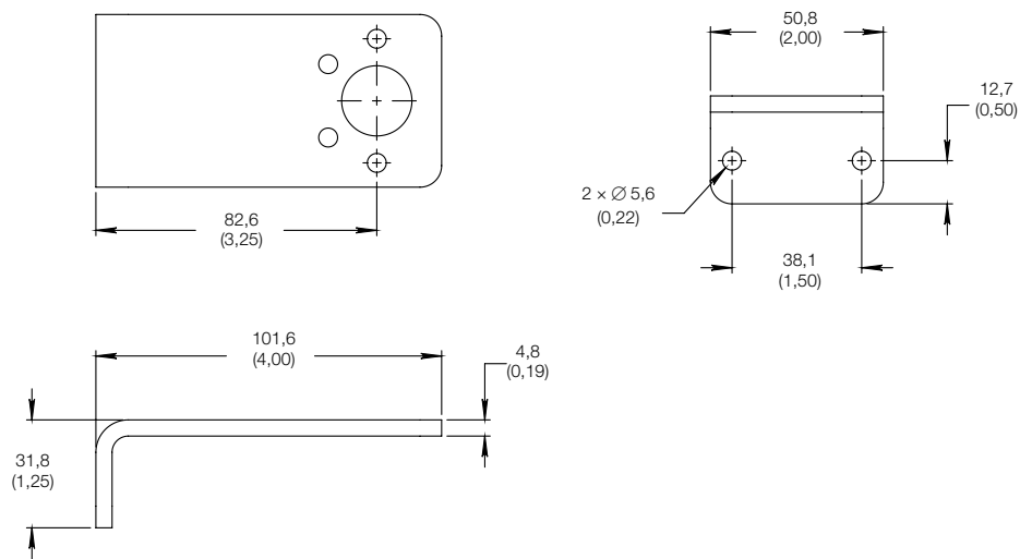
Support mural (Référence : 304-GSV-MBK-M)
